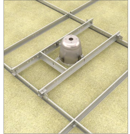
In het plenum zorgt een DLC clip voor extra ondersteuning van de verlichting.
