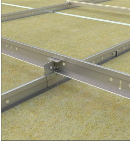
In het plenum wordt met de DLC clip een brug gevormd tussen obstakels in de ruimte.
