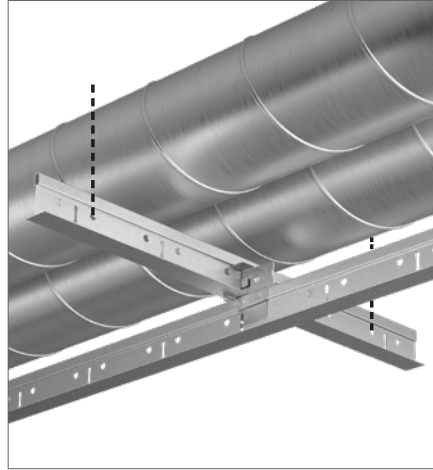
De DLC clip wordt gebruikt om een brug te maken onder het leidingwerk.
